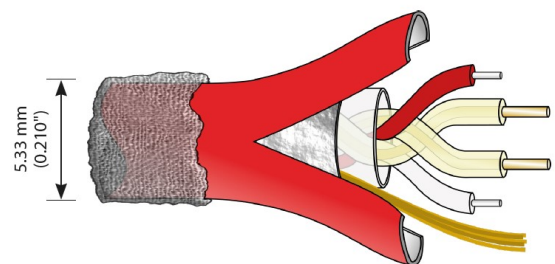
Rotes Sensorkabel mit Edelstahlgeflecht
