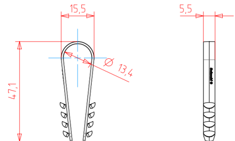
Dübelklemmschelle, Art.Nr. 22-11800-111
